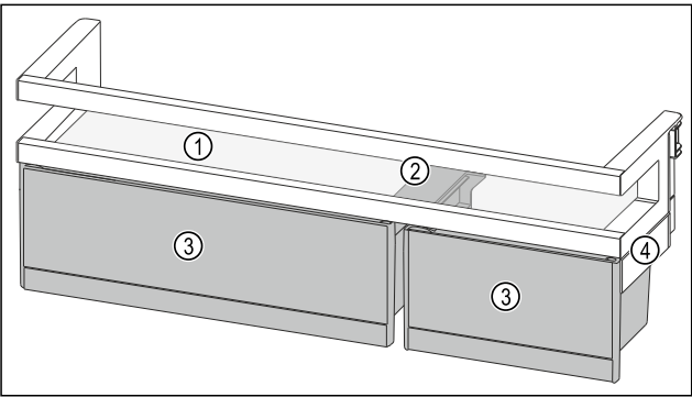
Fig. 79 Representación a modo de ejemplo del estante en la contrapuerta con VarioBoxes* (1) Estante (3) VarioBoxes (2) Pieza de retención para VarioBoxes (4) Parte lateral VarioBoxes
