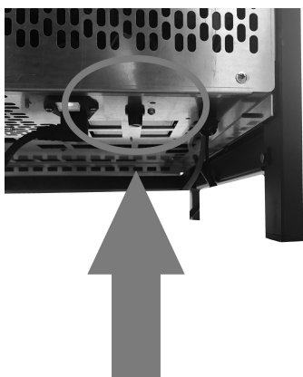
Fig. 23 - Rearme manual: debajo de la estufa FRAME³
