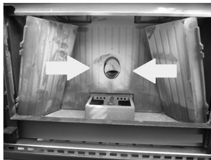
Fig. 33 - Extracción de las paredes laterales de hierro fundido
