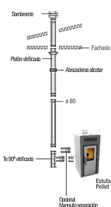
SALIDA VERTICAL CON TUBERÍA SIMPLE
