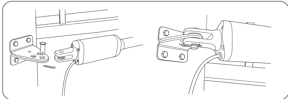
Montaje del motor en la pata del pilar
