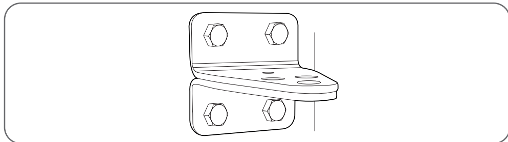
Montaje de la pata de la puerta al motor
