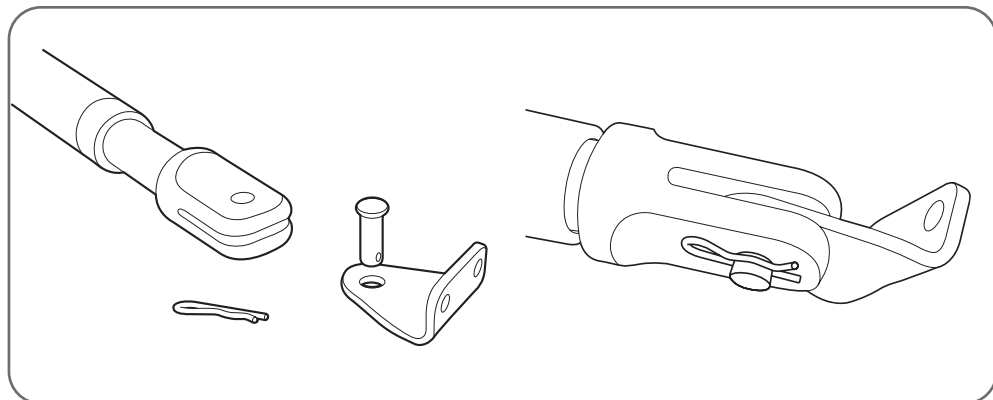
Montaje del motor en la pata del pilar
