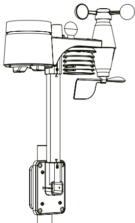
A. Montaggio su palo (Diametro 1"~1.3")(25~33 mm)
