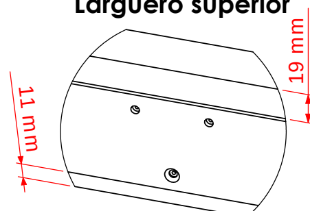
DETALLE B: Larguero superior
