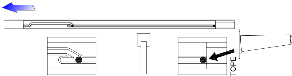
Acción 1: Elevar la barandilla para desbloquear el pivote superior hasta que el pivote inferior haga tope.
