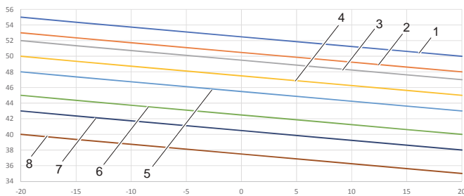
Modo calefacción (curva climática configurada H1)
