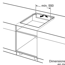
A: Profundidad de empotramiento
