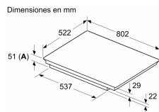
A: Profundidad de empotramiento
