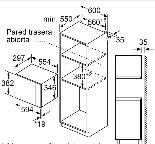
* 20 mm para frontal de metal Dimensiones en mm
