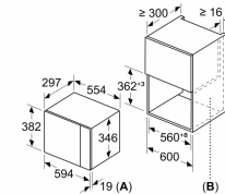
A: 20 mm para frontal de metal B: Pared trasera abierta
