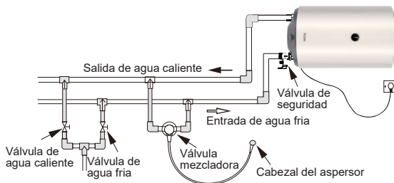
Figura 3 Diagrama de Instalación - Instalación Horizontal deberá ser llevado a cabo en base al diagrama
