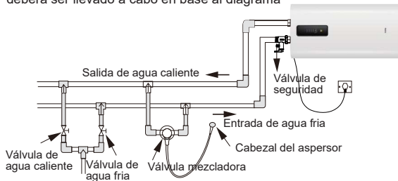
Figura 3 Diagrama de Instalación - Instalación Horizontal (serie TF7/TF7W/VH1/VH3W)
