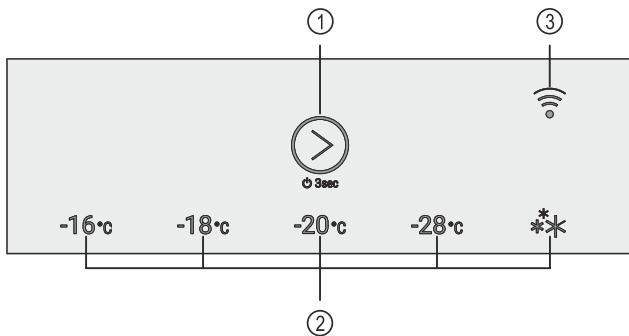
Fig. 23 Elementos de manejo y de indicación
