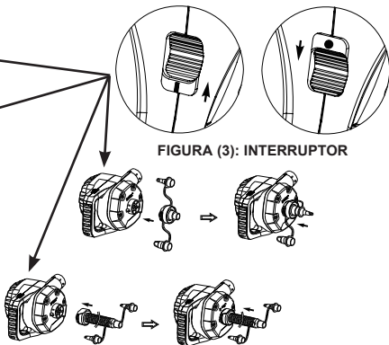
FIGURA (4): CONECTE EL BOQUILLA O SUJETAR LA MANGUERA
