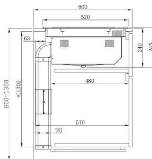
Odváděcí varianta
