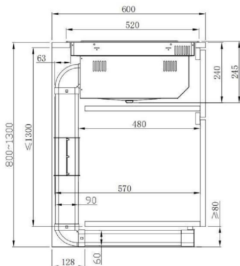
Filtrerande version
