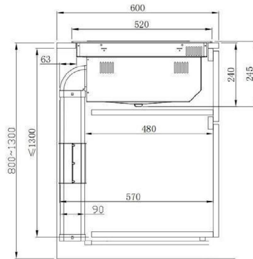
Avtrekksversion
