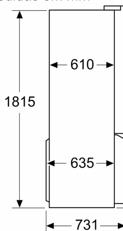
Medidas em mm
