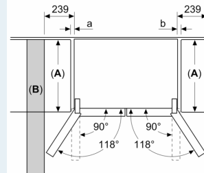
Medidas em mm
